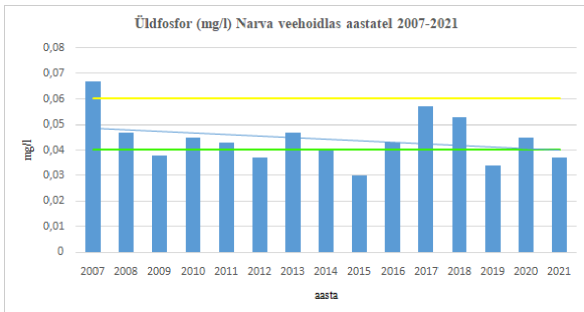
Joonis 4. Narva veehoidla keskmised üldfosfori sisaldused aastatel 2007-2021
