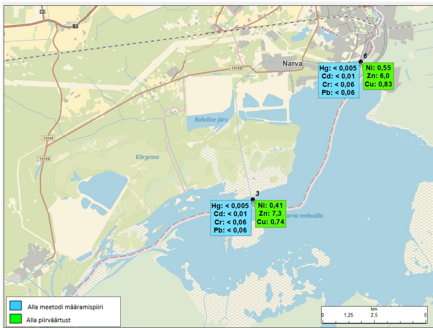
Joonis 5. Raskmetallide sisaldused (µg/l) Narva veehoidlas 2021. aasta augustis
