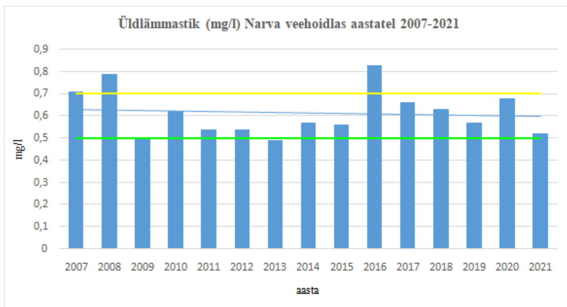
Joonis 3. Narva veehoidla keskmised üldlämmastiku sisaldused aastatel 2007-2021
