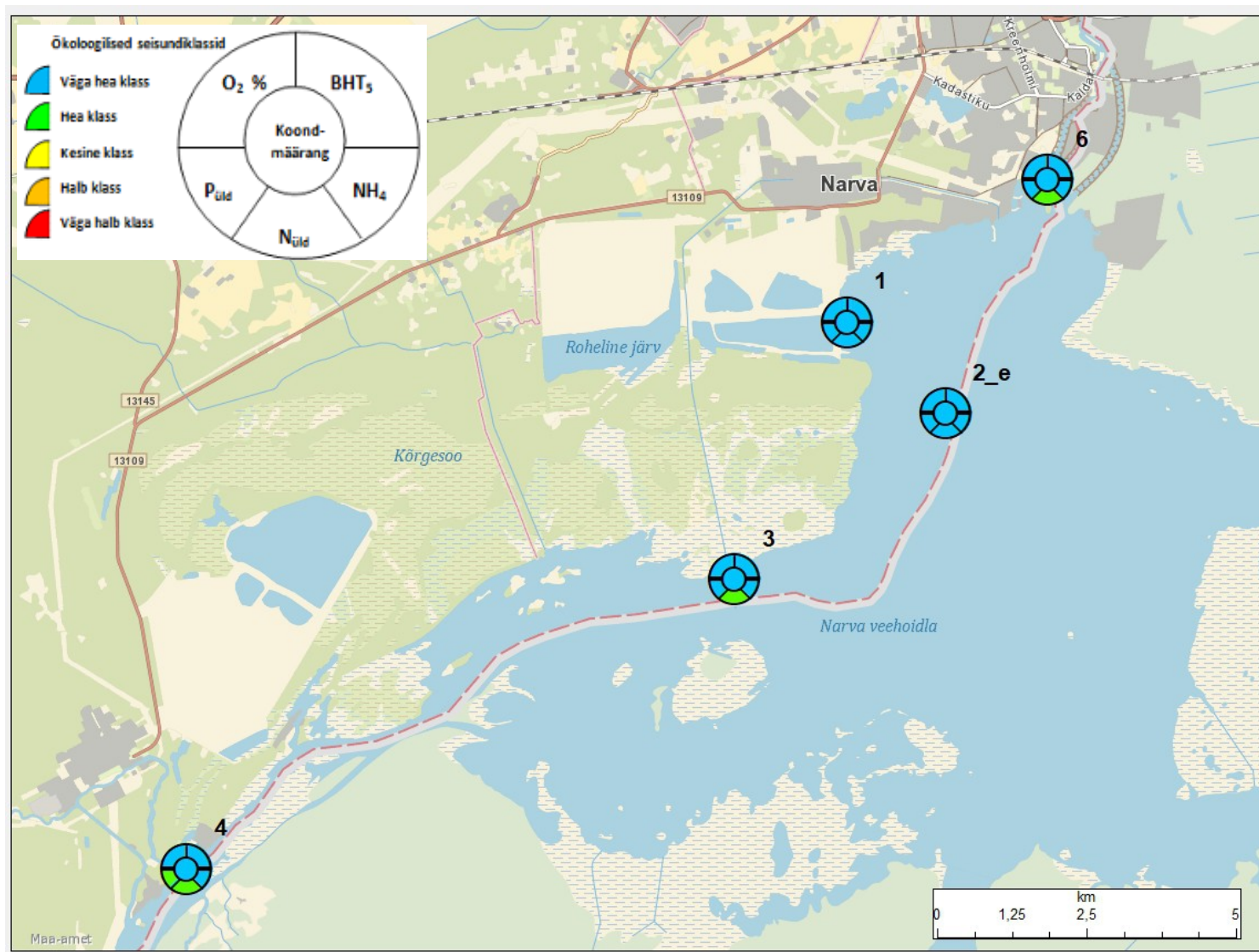
Joonis 2. Narva veehoidla füüsikalise-keemiliste kvaliteedinäitajate ökoloogilised seisundiklassid ja koondmäärangud 2021. aasta augustis
