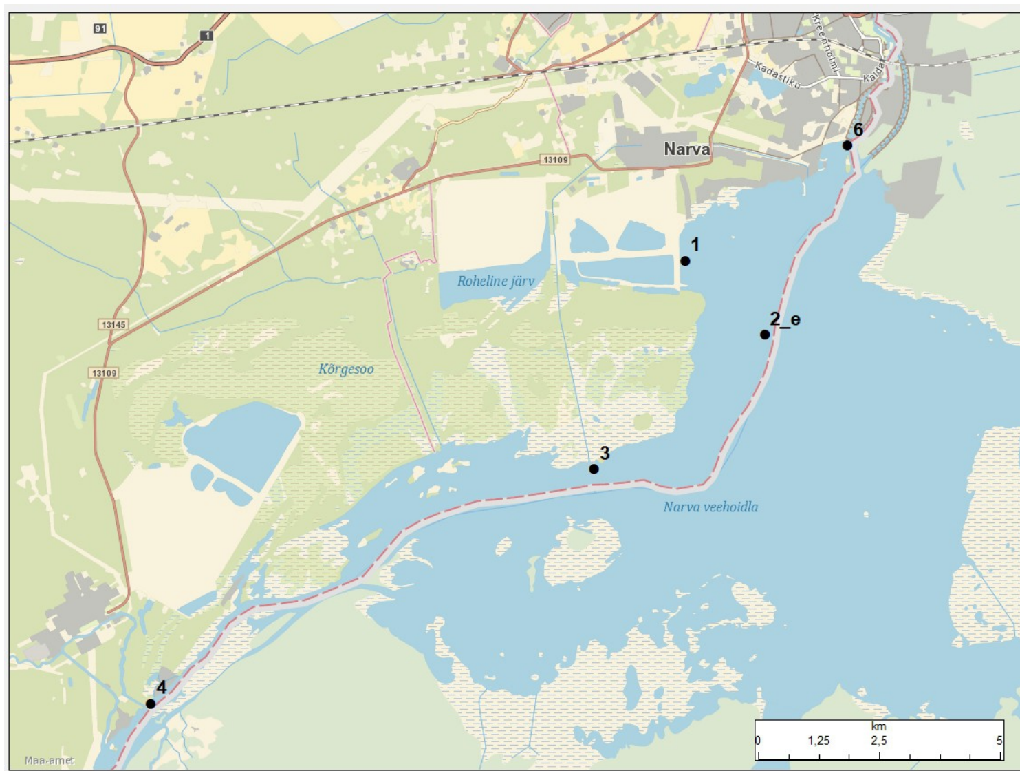
Joonis 1. Seirejaamade asukohad Narva veehoidlal 2021. aastal
